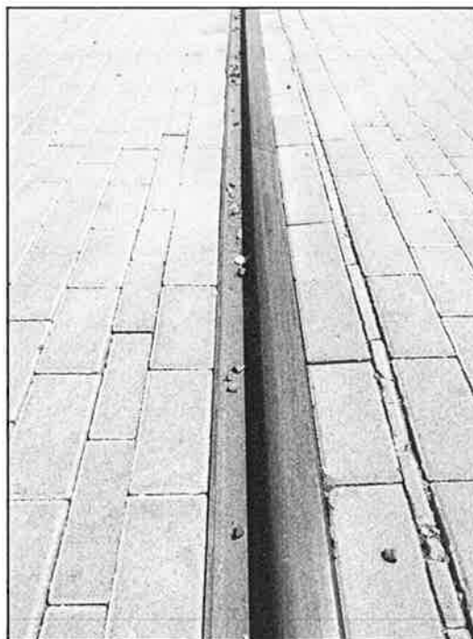
Zdj. 11 Przykład ogranicznika stalowego przy szynie
