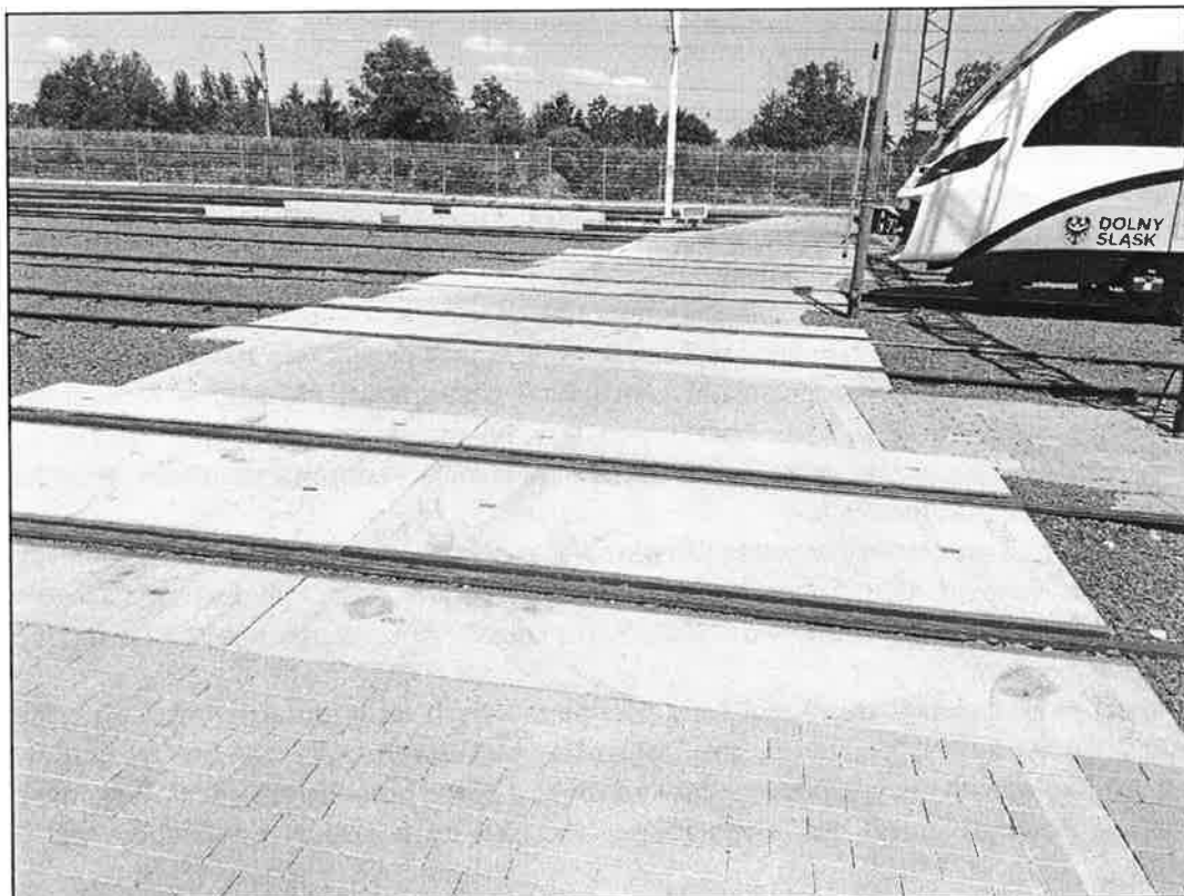
Zdj. 9 Przykład przejścia przez tory – oczekiwania zamawiającego
