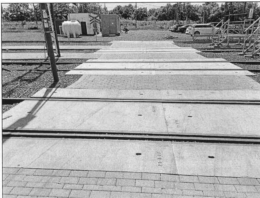
Zdj. 10 Przykład przejścia przez tory – oczekiwania zamawiającego
